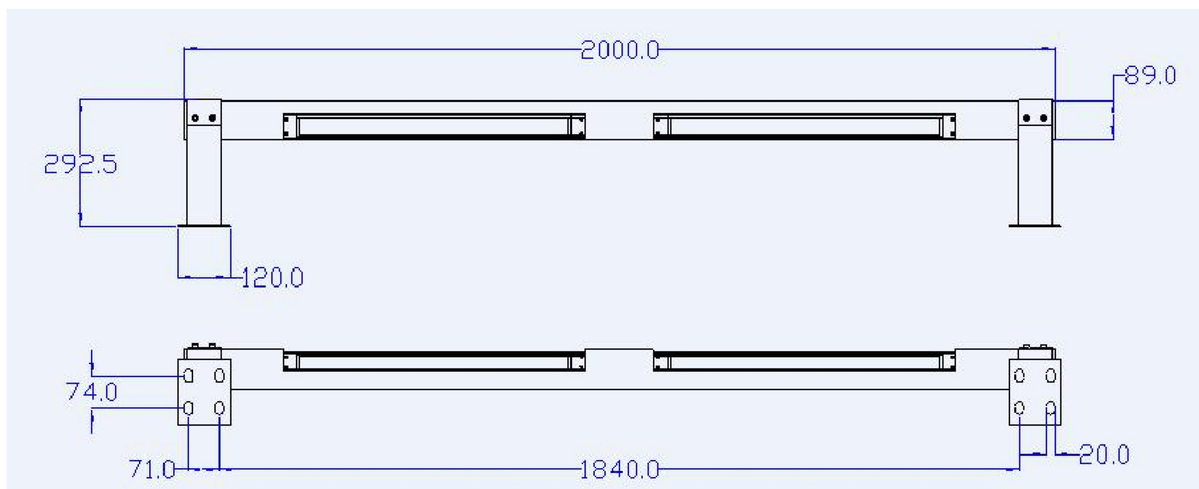
直径 89 管尺寸图：
